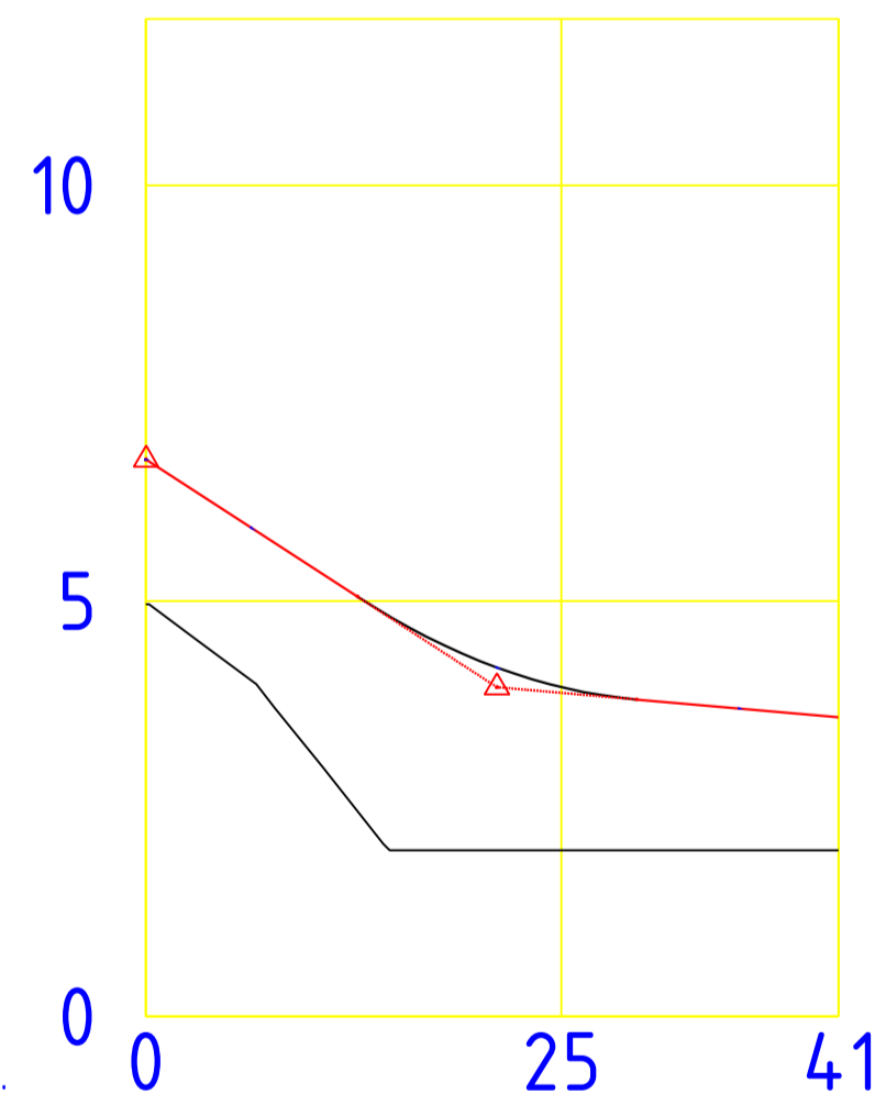
PROFIL: Veglinje 3 H.O.H SKALA L= 500 H= 100
