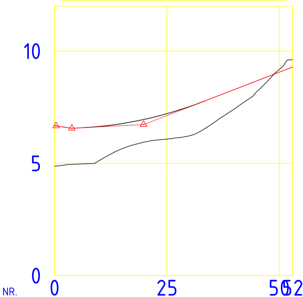
PROFIL: Veglinje 2 H.O.H SKALA L= 500 H= 100
